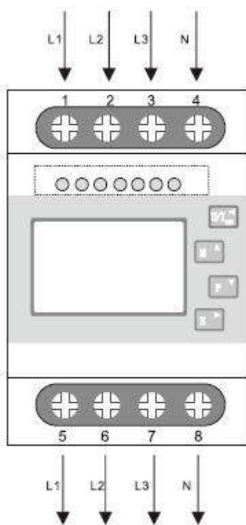
三相四线
