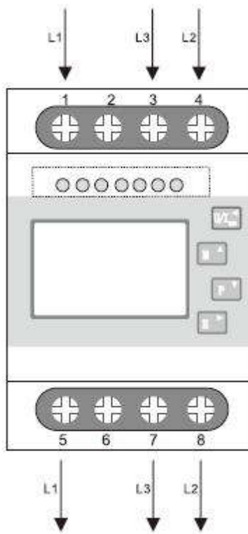
三相三线
